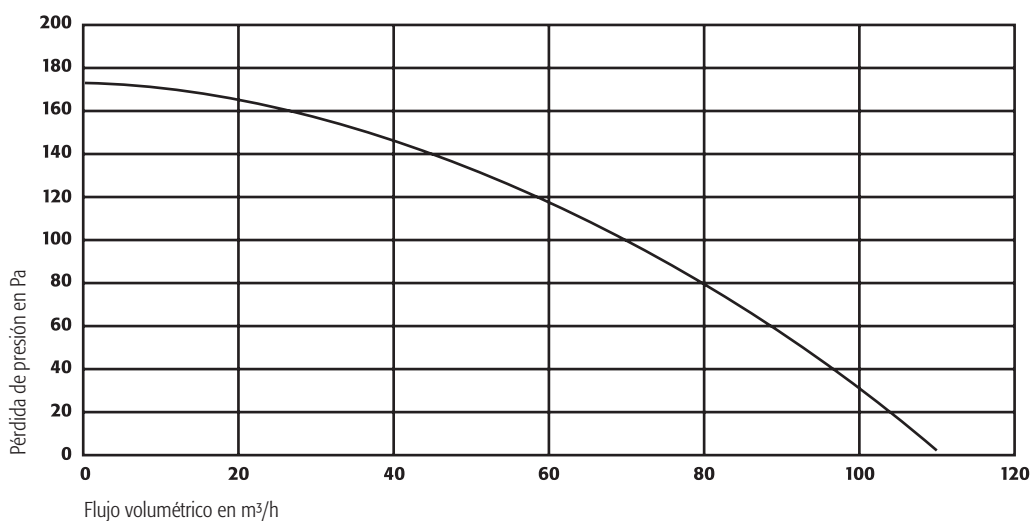
Curva característica
